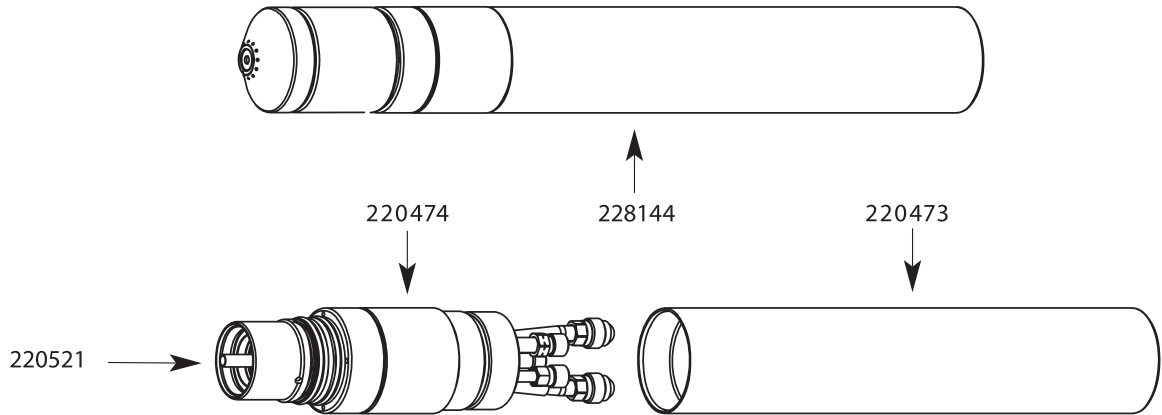
HYPERFORMANCE PLASMA HSD130 - TORÇ MONTAJ SEÇENEKLERİ
